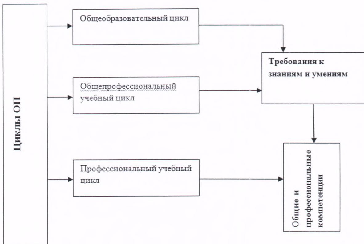
Рисунок 2 – Циклы ППКРС
